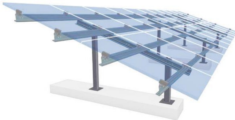
Kuva 3-3. Esimerkkikuva maavaraisesta painovoimaan perustuvasta perustustavasta.
